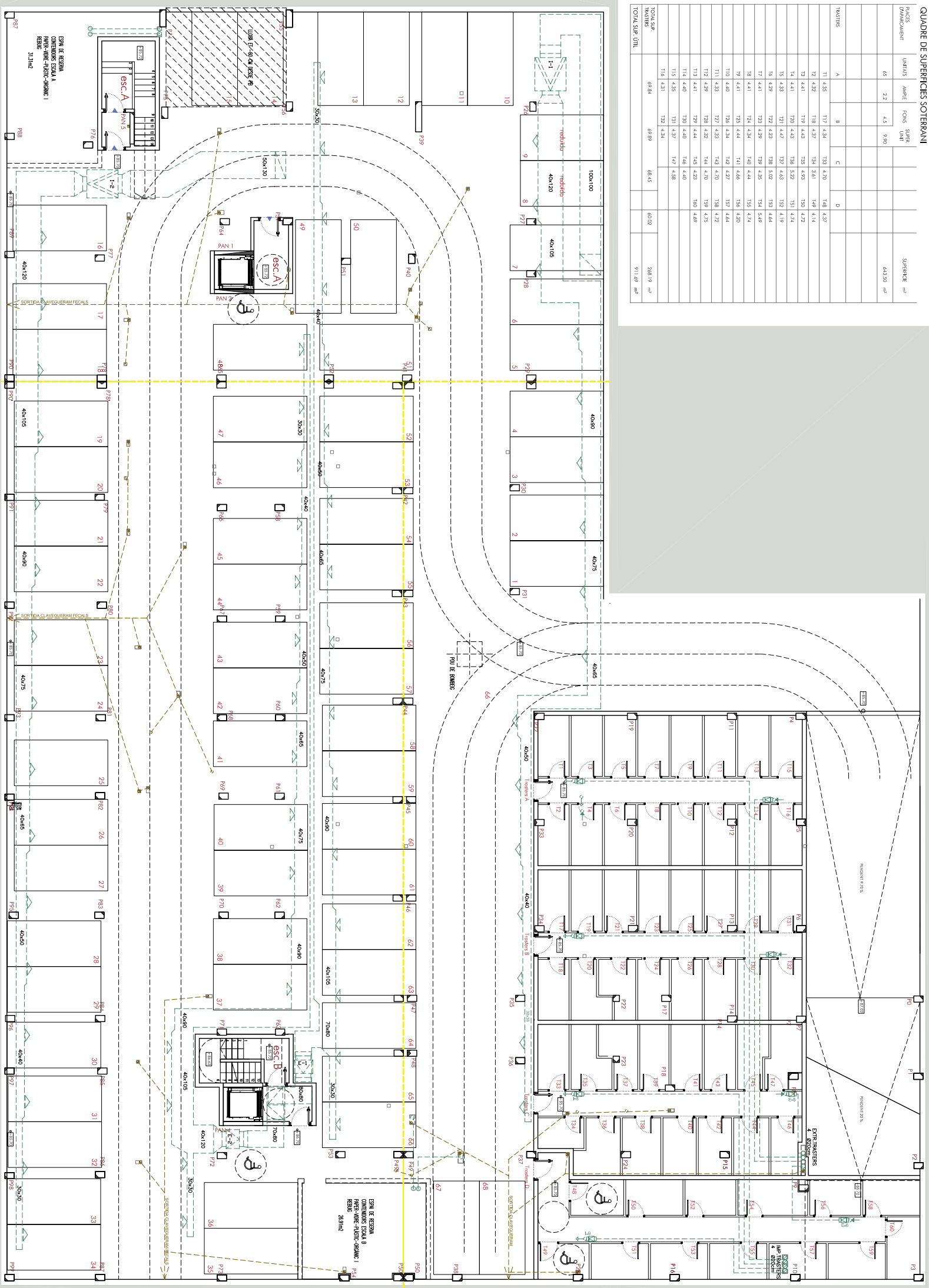
PLANTA SOTERRANI
